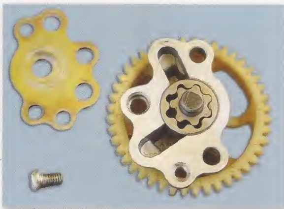
Ensamble de bomba trocoidal
